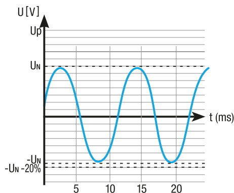
Señal con voltaje normal
