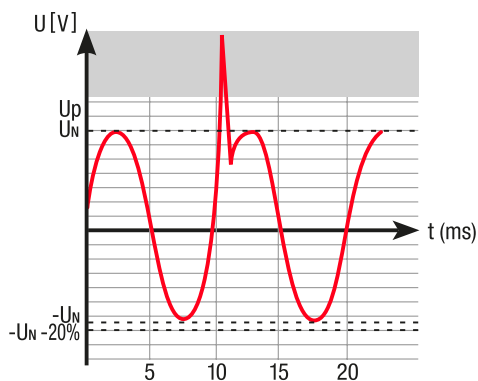
Señal con pico de voltaje
